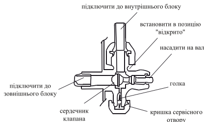
Схема 3-ходового клапана
